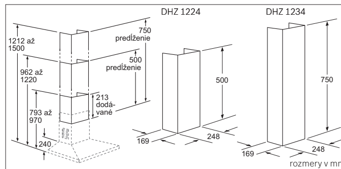
Predĺženie komína DHZ 1224 | 1234
