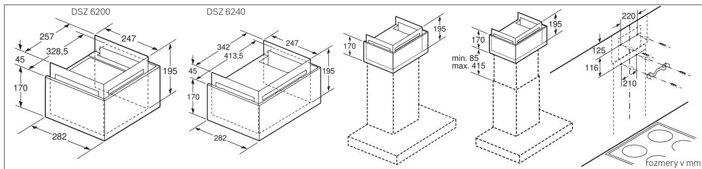
Modul CleanAir pre komínové odsávače DSZ 6200 | DSZ 6240
