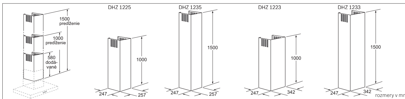
Predĺženie komína DHZ 1225 | 1235 | 1223 | 1233
