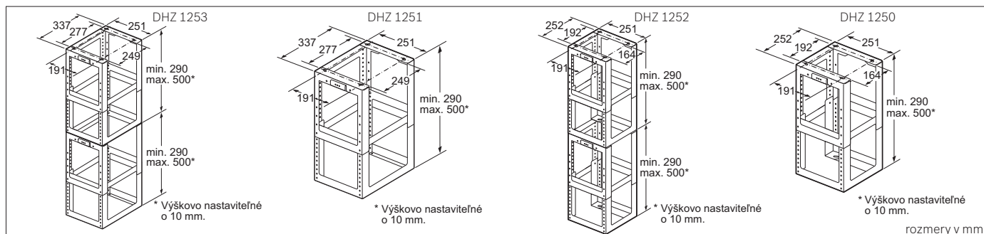
Konštrukcia na predĺženie komína DHZ 1253 | 1251 | 1252 | 1250
