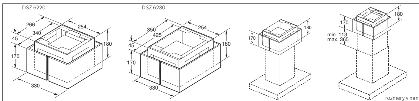
Modul CleanAir pre ostrovčekové odsávače DSZ 6220 | 6230
